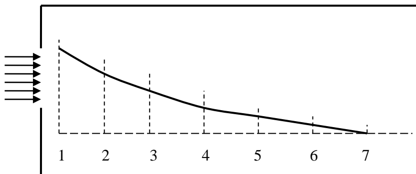
Рис. 9. Расположение точек замера и кривая изменения КЕО в поперечном разрезе помещения с односторонним боковым освещением
