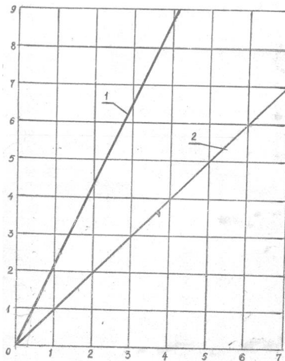
Рис. 17. Тарировочный график: 1 – АСО-3; 2 – чашечный анемометр
