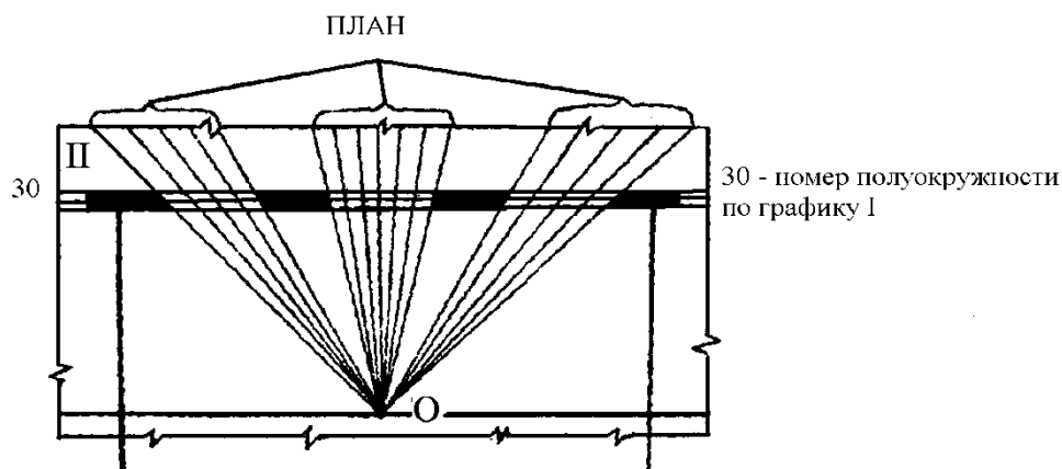
Рис. 6. Определение количества лучей n_1 и n_2 , проходящих через световые проемы в стене при боковом освещении, по графику II
