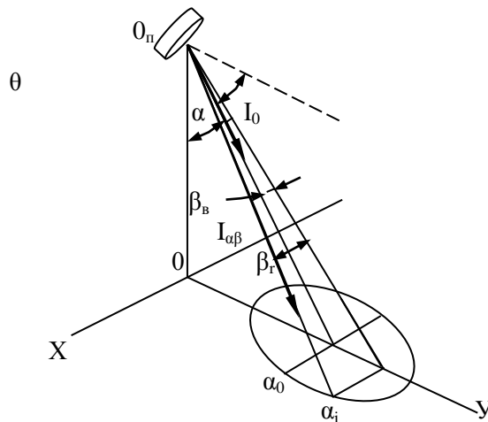
Рис. 3. Схема для расчета освещенности, создаваемой прожектором
