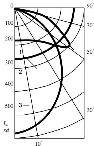
Рис. 2. Кривые распределения силы света в пространстве: 1 – широкая; 2 – равномерная; 3 – глубокая
