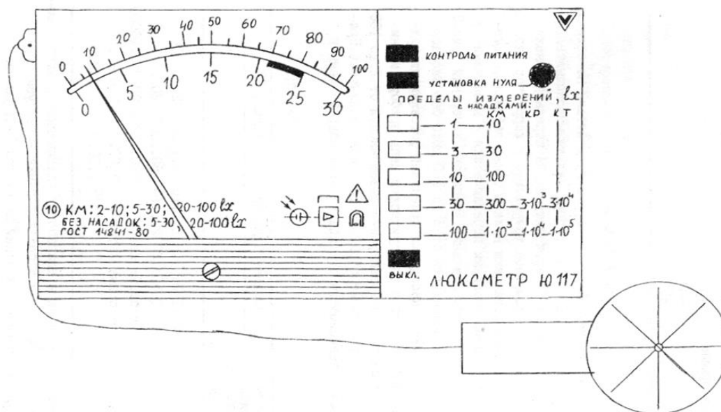
Рис. 8. Люксметр Ю-117
