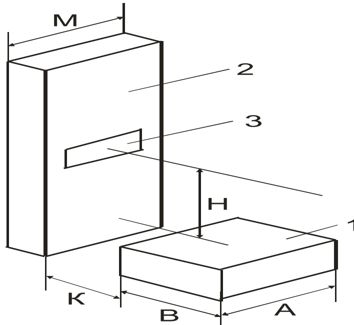
Рис. 19. Устройство односторонней отсасывающей панели: 1 – источник вредных выделений; 2 – односторонняя панель; 3 – всасывающее отверстие панели
