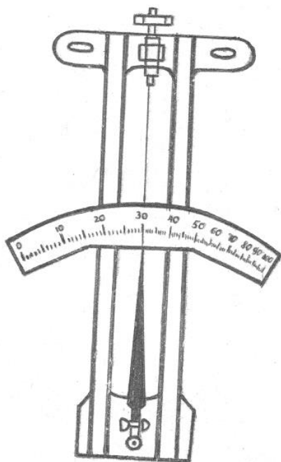
Рис. 12. Гигрометр М-19
