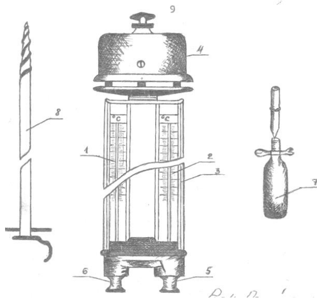
Рис. 13. Психрометр Ассмана
