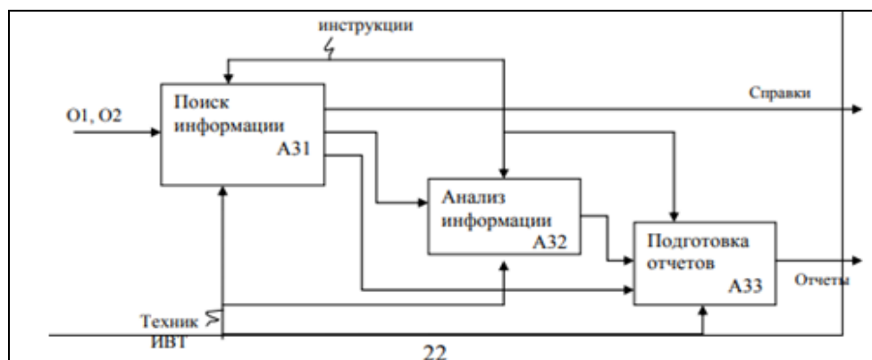
Рисунок 8 - Диаграмма процесса «Подготовка справок и отчетов»
