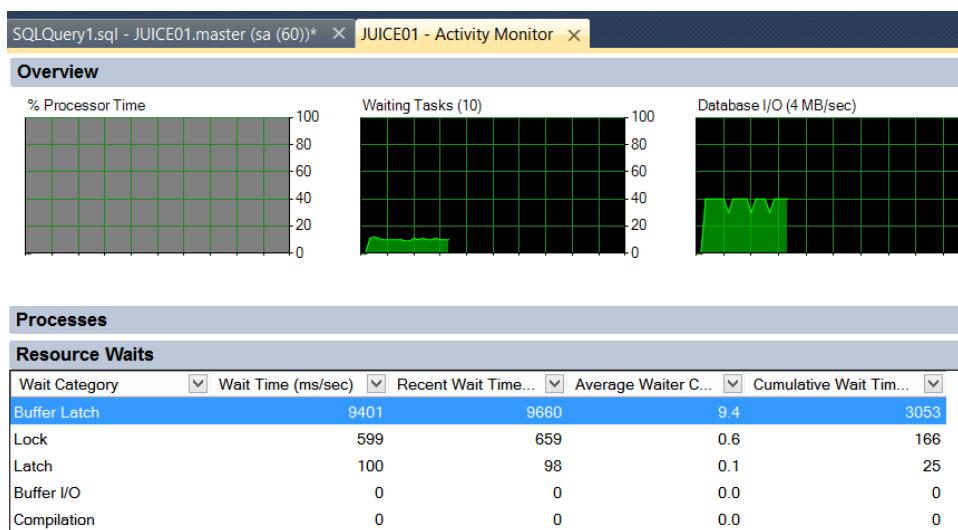
Рисунок 10 – Монитор действий
