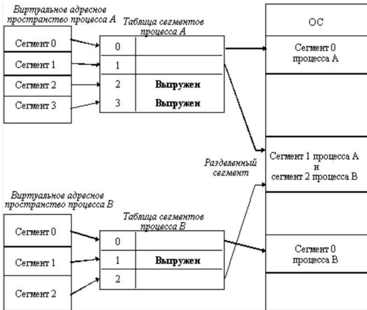
Рисунок 14 – Распределение памяти сегментами
