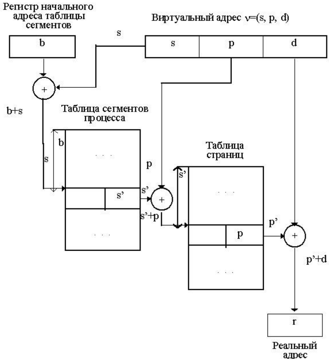
Рисунок 21 – Преобразование виртуального адреса при странично-сегментной организации
