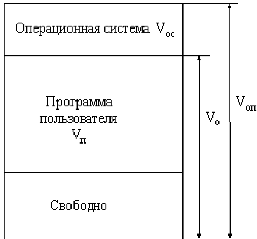
Рисунок 17 – Организация памяти при связном распределении для одного пользователя
