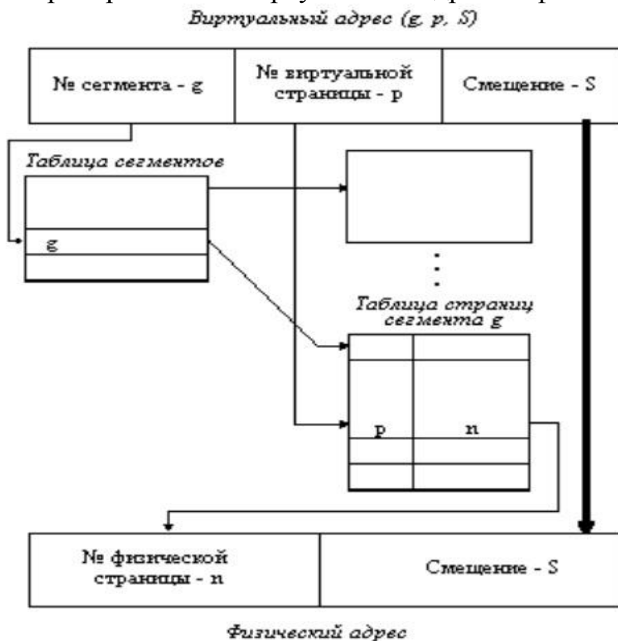
Рисунок 15 – Схема преобразования виртуального адреса в физический для сегментно-страничной организации памяти
