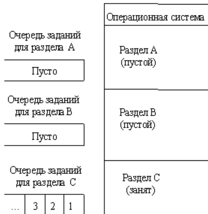
Неэффективное использование памяти при распределении фиксированными разделами
