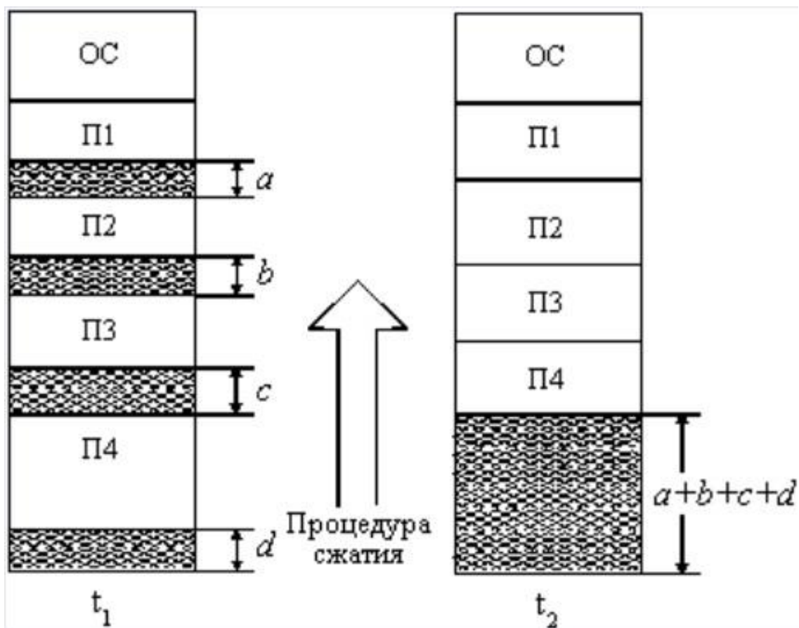
Рисунок 11 – Распределение памяти перемещаемыми разделами
