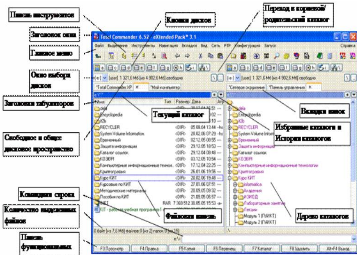
Рисунок 26 – Окно файлового менеджера Total Commander
