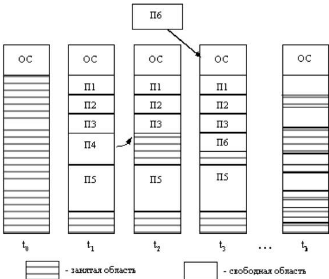
Рисунок 10 – Распределение памяти динамическими разделами
