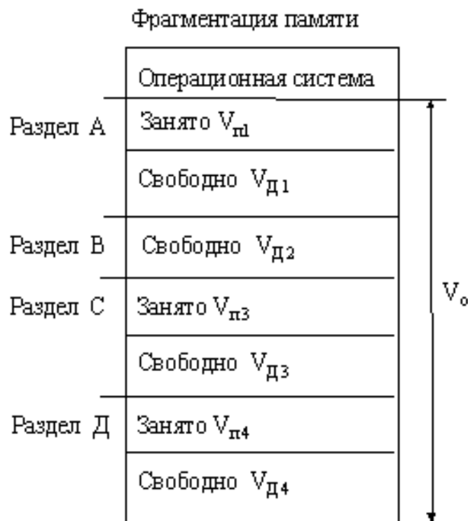
Рисунок 19 – Фрагментации оперативной памяти
