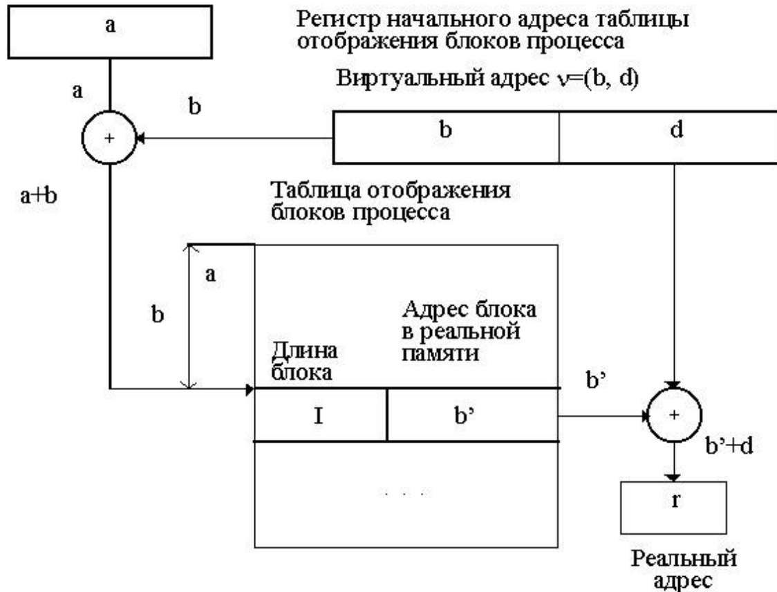
Рисунок 20 – Преобразование виртуального адреса
