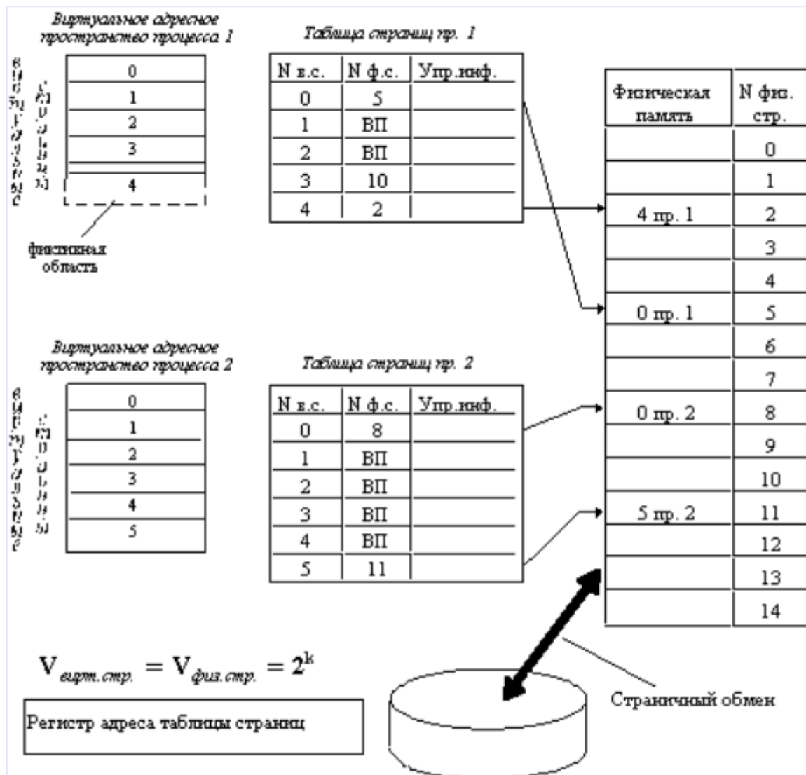
Рисунок 12 – Страничное распределение памяти
